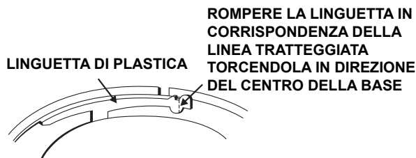
Figura 3a: Attivazione della funzione antimanomissione
