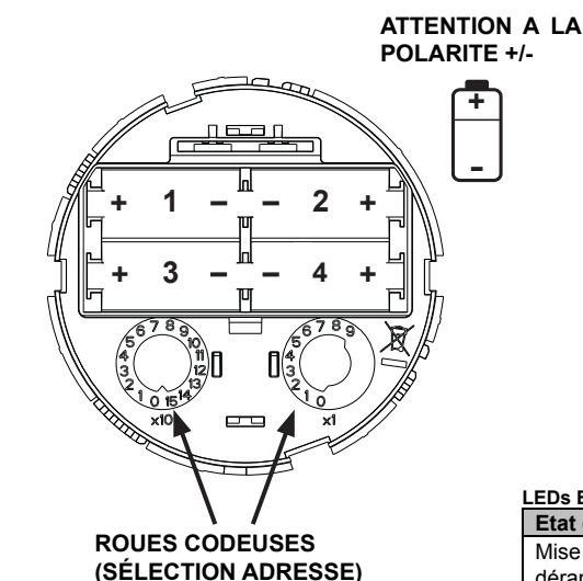
Figure 4: Installation des piles et Roues Codeuses
