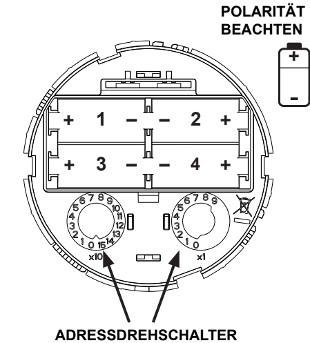
Abbildung 4: Batterieinstallation und Adressdreheschalter
