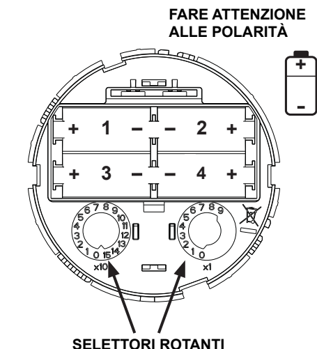
Figura 4: Alloggiamento delle batterie e selettori rotanti per l'indirizzamento
