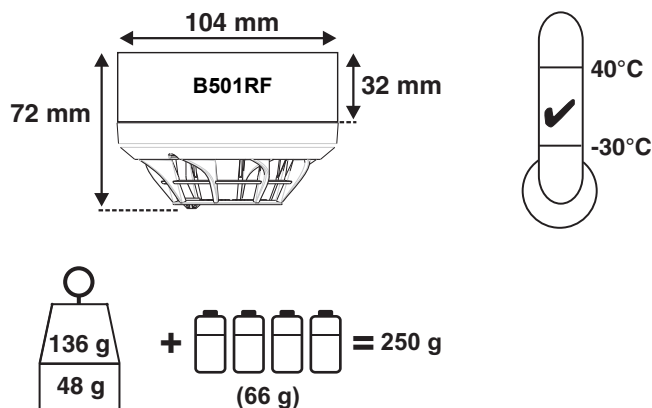
Figura 1: Montaggio B501RF
