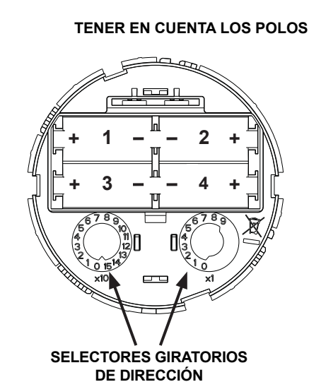
Figura 4: Instalación de las pilas y Selectores giratorios de dirección
