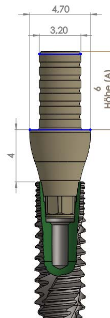
Meoplast mit Heilkappe (Maße in mm)
